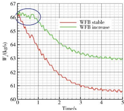
图16 进气道出口流量随时间变化曲线
