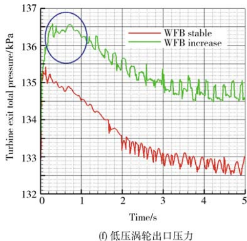
图 17 发动机工作参数随时间的变化
