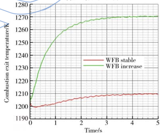
(d) 涡轮前温度
