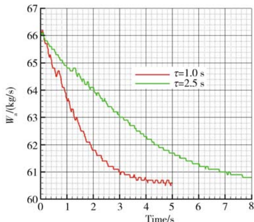
图 11 进口截面气流流量随时间变化曲线
