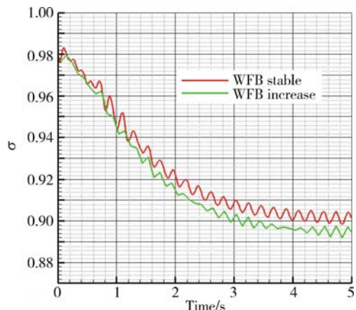
图 15 总压恢复系数随时间变化曲线
