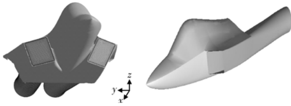
图 5 前机身/进气道一体化模型 Fig. 5 Aeroplane forebody/air inlet integrated model
