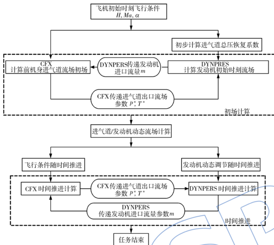
图2 程序运行时流程图
