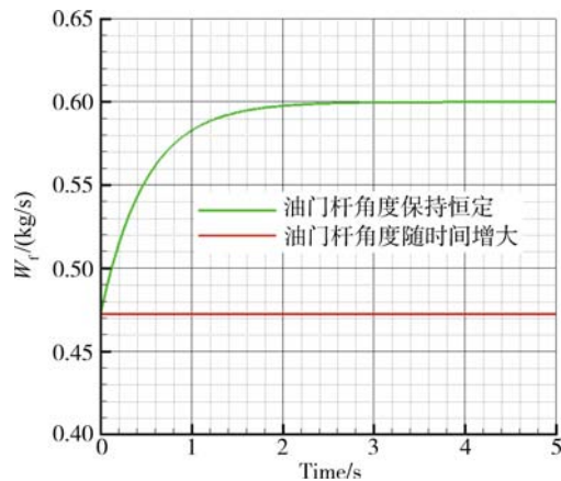
图 13 发动机燃油流量随时间变化
