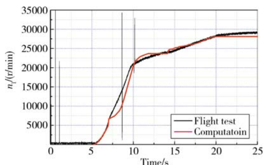
图4 低压转速随时间变化结果对比
