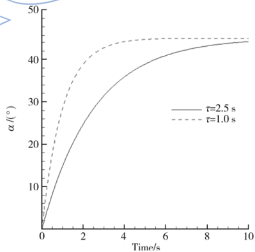
图 7 \tau=1.0\text{ s} 和 \tau=2.5\text{ s} 攻角 \alpha 随时间变化
