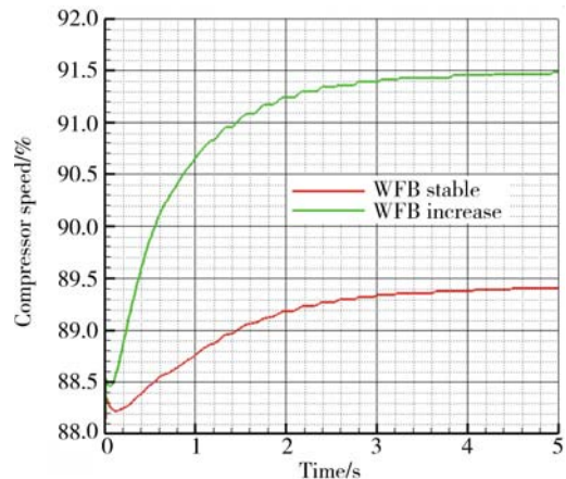
(b) 高压转速
