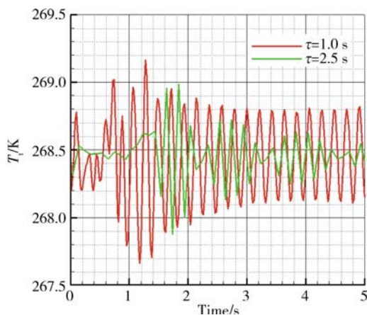
图8 出口平均总温 T_t 的时间曲线
