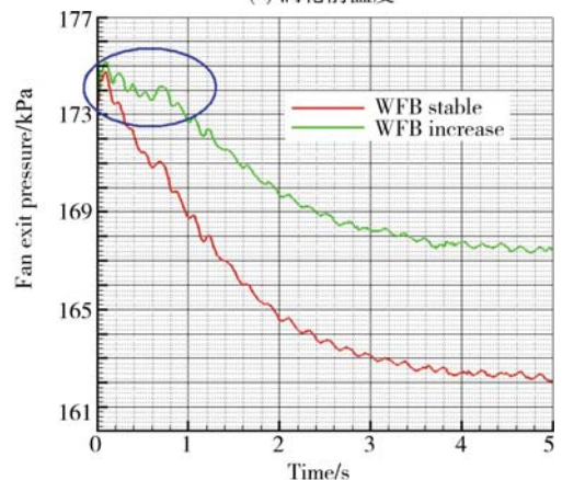
(e) 风扇出口压力
